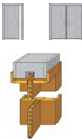
Schiebetürzargen in der Wand laufend Sliding door frame inside the wall opening
