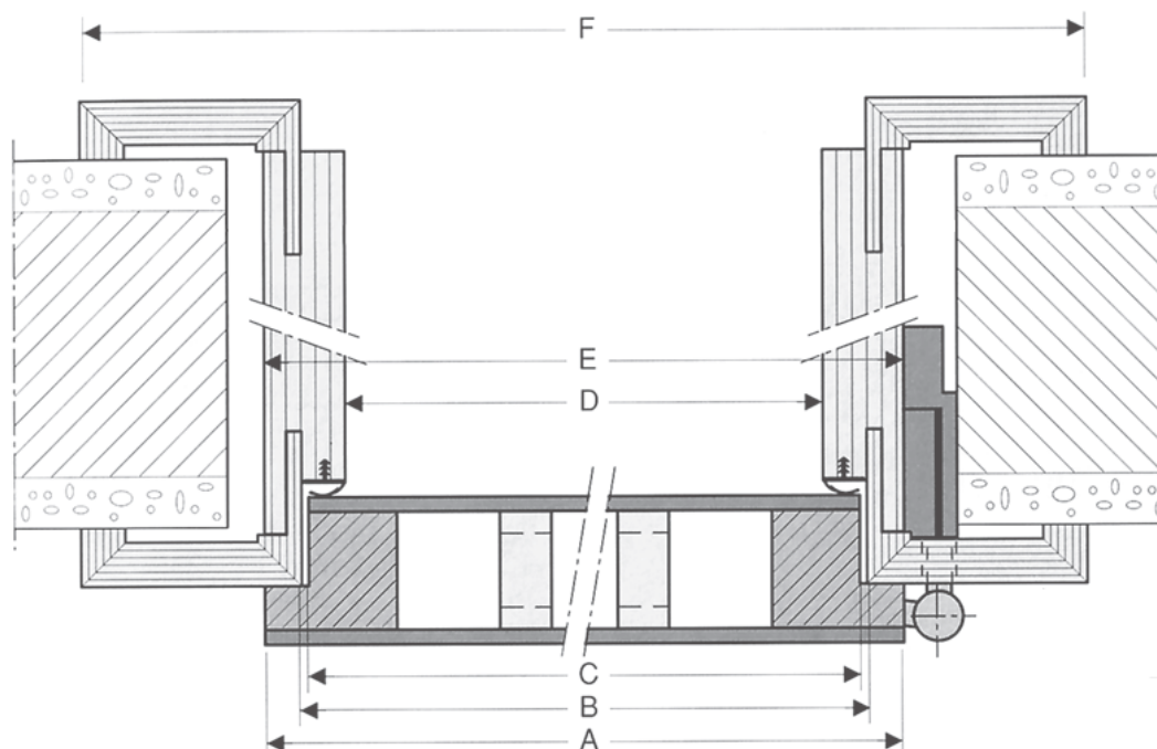
Maßtabelle DIN / Dimension table DIN
