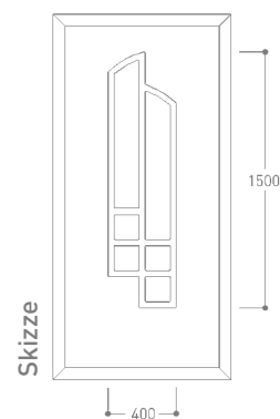
Detail Favorit 10 mit Sandstrahlglas Y 866 Float
