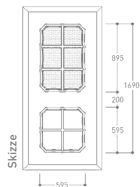
Detail Direkt 6 Ornamentrahmen
